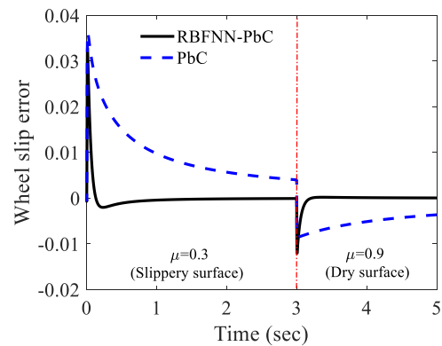
شکل ۸-الف: مقایسه عملکردهای RBFNN-PbC و PbC در مانور ۳،
