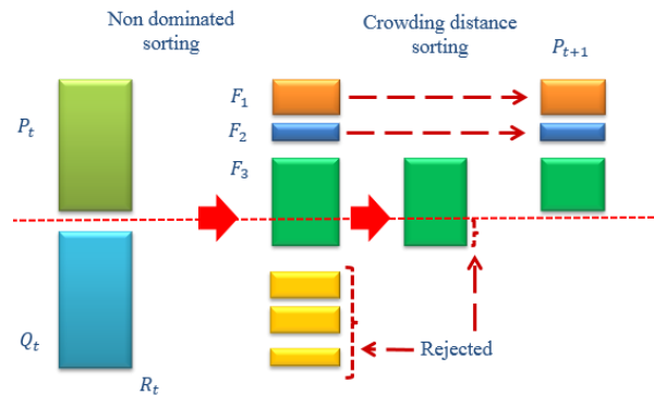
شکل ۳: مراحل کار NSGA-II [۴۵]
