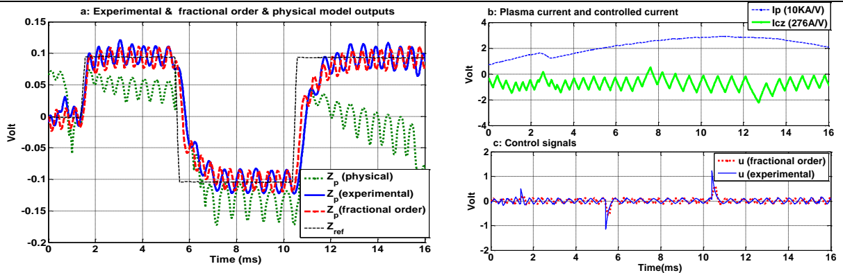
شکل ۱۷: a- مکان عمودی پلاسما برای شات ۲۲. b- جریان پلاسما ( I_p )، جریان کنترلی (I_{cz}) ، c- سیگنال کنترلی عملی و حالت شبیه سازی با مدل کسری
