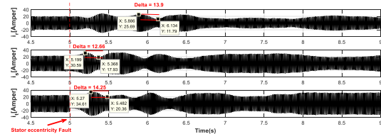
شکل ۹- بزرگنمایی شده جریان های تغذیه موتور القایی در شرایط عیب سناریوی اول
