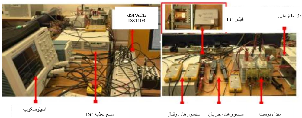
شکل ۸- میز آزمایشگاهی.
