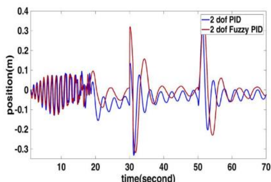
شکل ۸: عملکرد کنترل کننده ها در پایداری سازی موقعیت ارباب (swing up به همراه اغتشاشات خارجی)
