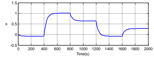
شکل (۱۲): نتایج ردیابی کنترل کننده مقاوم برای دستگاه CSTR
