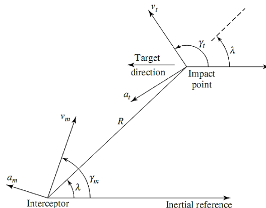
شکل ۳: هندسه ی دوبعدی درگیری موشک و هدف [۱۴]
