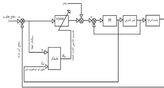
شکل ۳: ساختار سیستم کنترل پیشنهادی سطح آب درام
